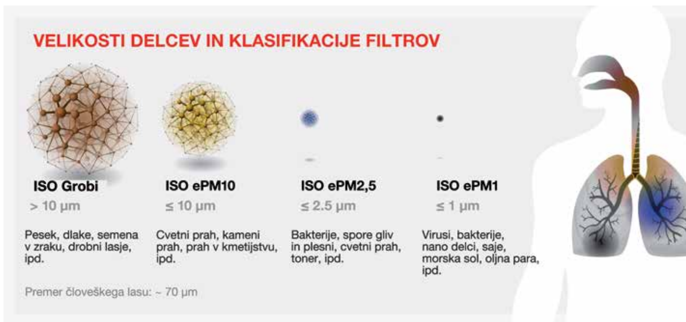
Velikosti delcev in klasifikacija filtrov po novem standardu ISO 16890 za zračne filtre
